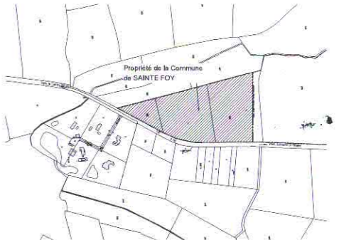
EXTRAIT CADASTRAL Etoile 10000 RD 109 - "La Jassière" 85150 SAINTE FOY SECTION 9 N°386-388 SUPERFICIE 30248 m² LIMITE PARCELLAIRE
